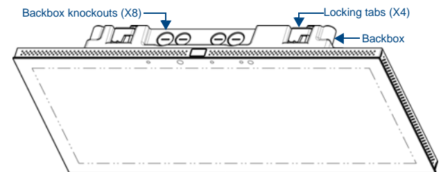
FIG. 3 MXD-2001-PAN (Landscape)
