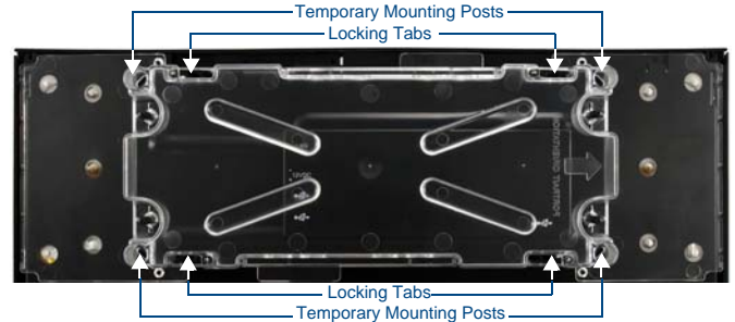
FIG. 2 MXD-2001-PAN Backbox
