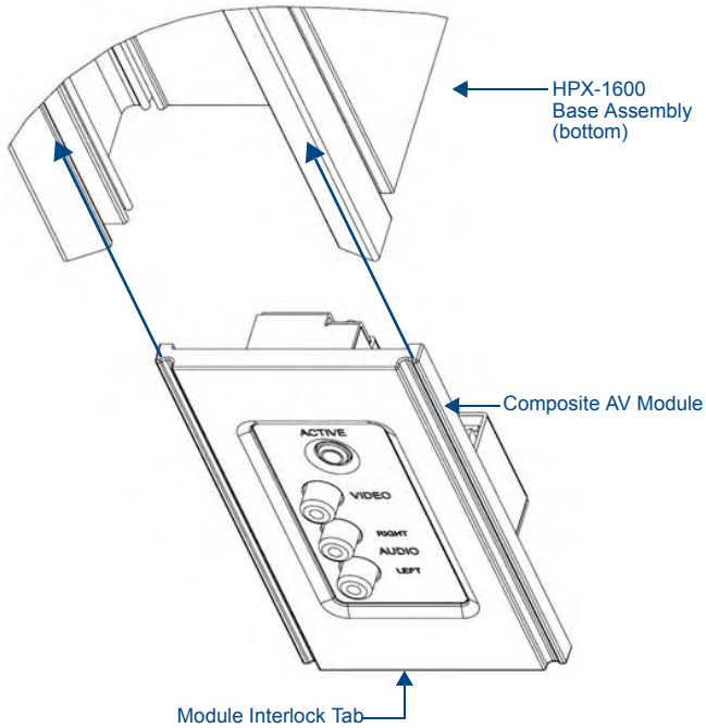
FIG. 6 Inserting the Composite AV Module into the HPX-1600 Chassis
