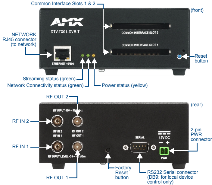
FIG. 1 DTV-TX01-DVB-T Transmitter
